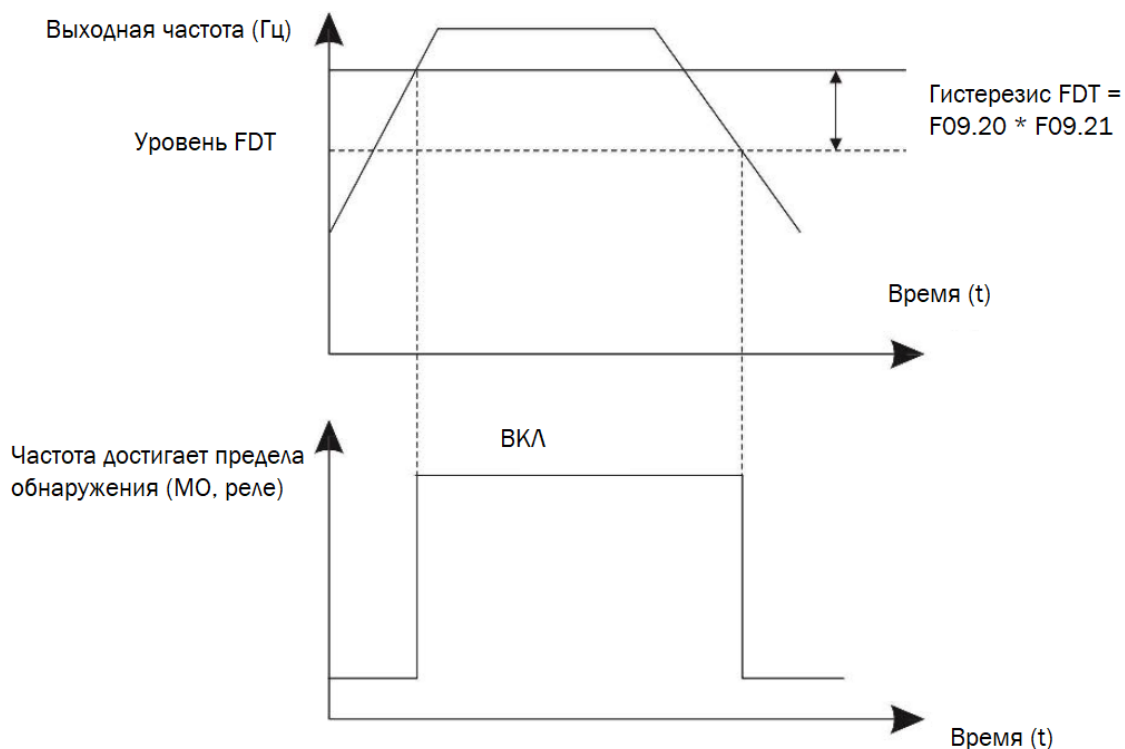
Рисунок 6-15 – Функция FDT
